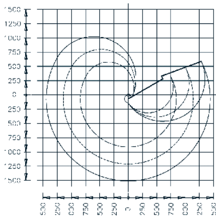
Planimetria Braccio SX
